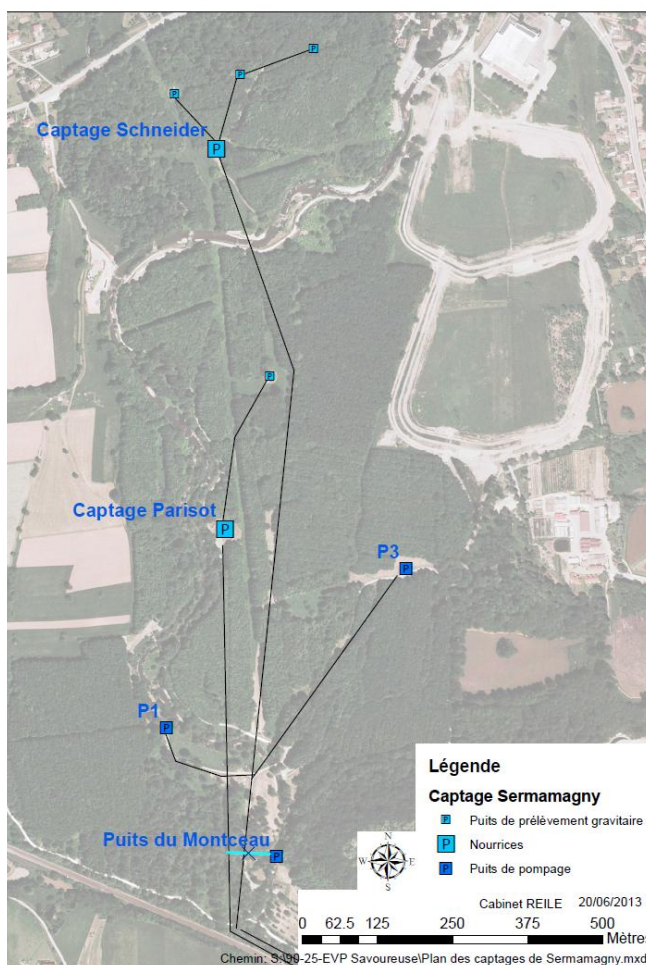
Carte 5 : plan du champ captant de Sermamagny
