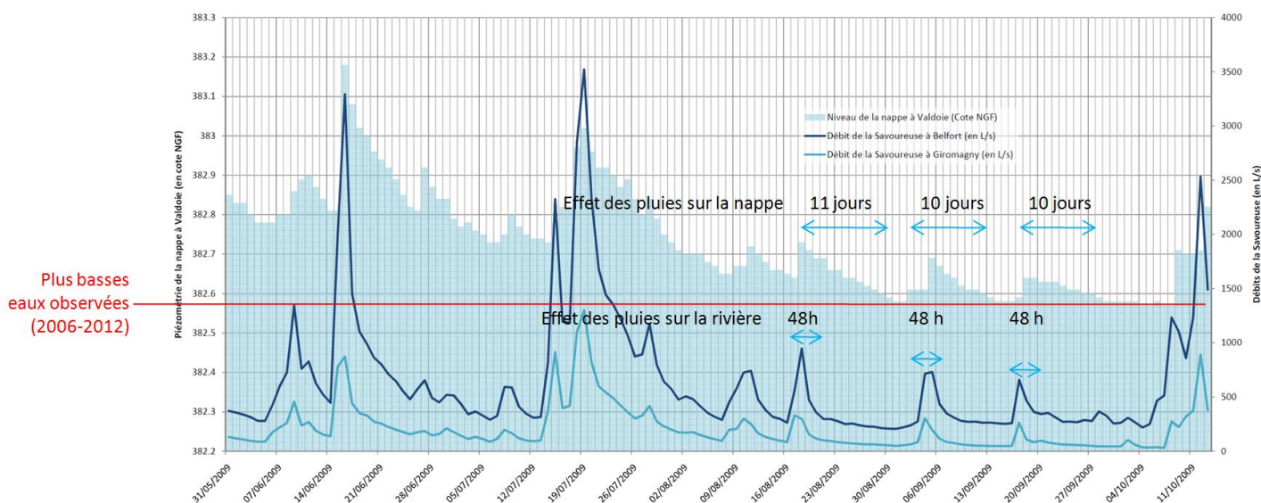
Graphes N° 2 et 3 : Détail des variations de débits de la Savoureuse et des variations de la piézométrie à Valdoie lors de l'été 2009
