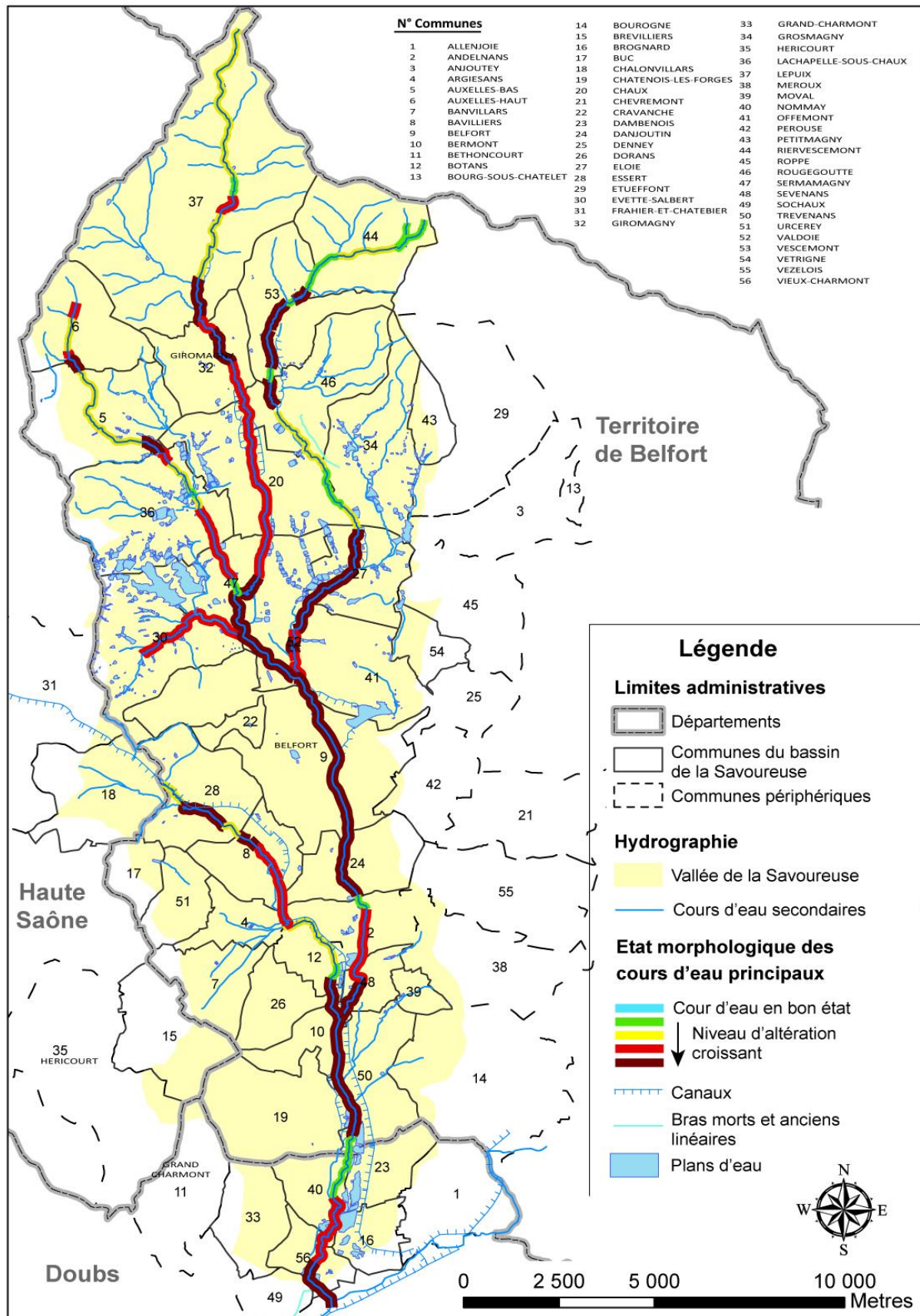
Carte 2 : Etat physique des cours d'eau de la vallée de la Savoureuse (rappel) Origine des données : ONEMA
