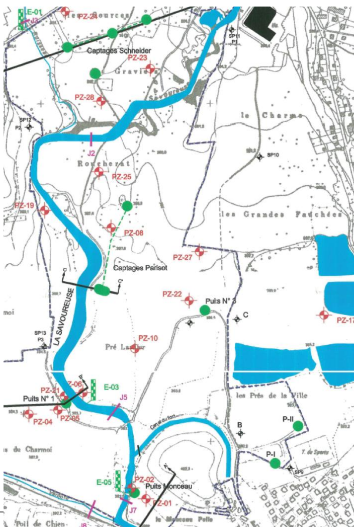
Carte 7 : Localisation des piézomètres du champ captant de Sermamagny
